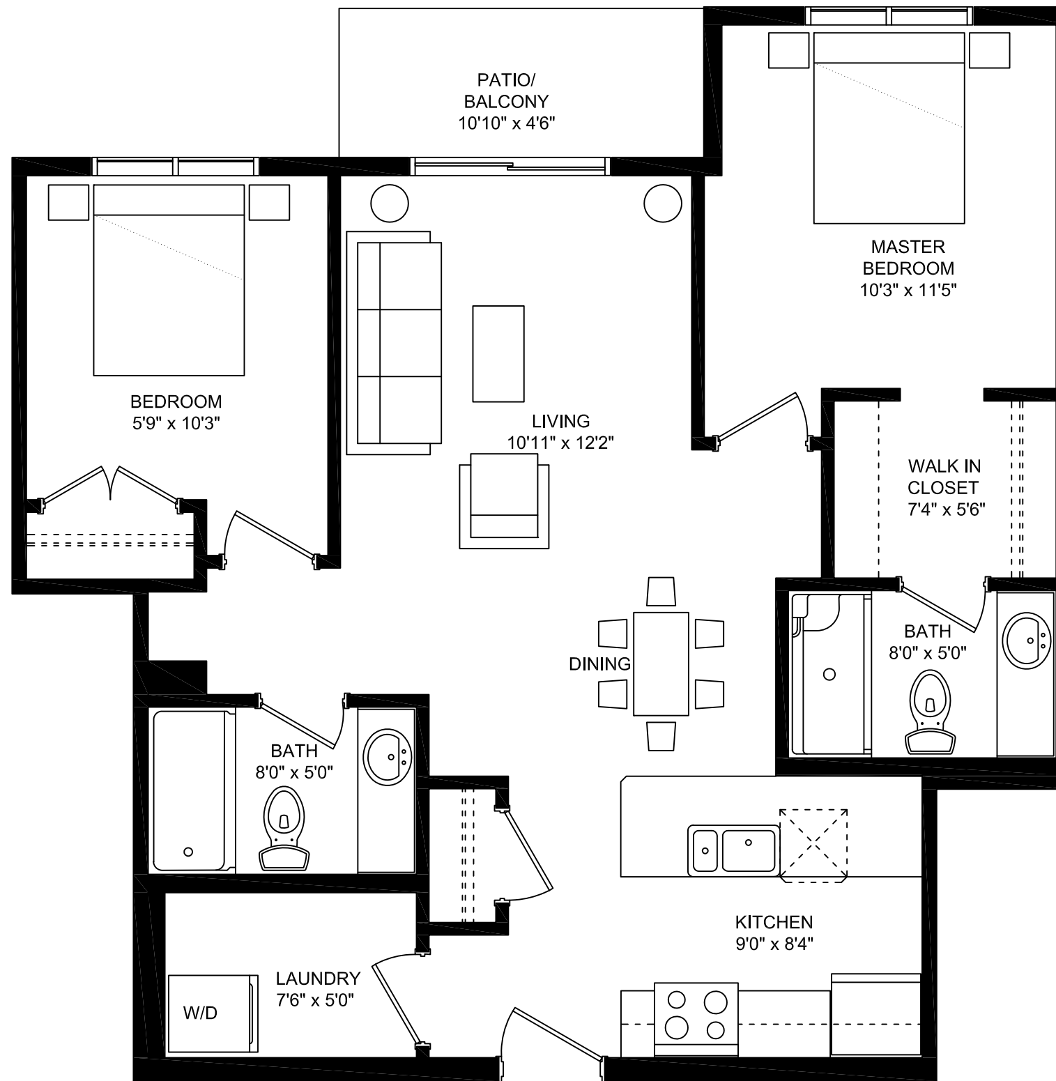
PLAN: UNIT A - 761 SFT Scale: 1/4" - 1'0"
