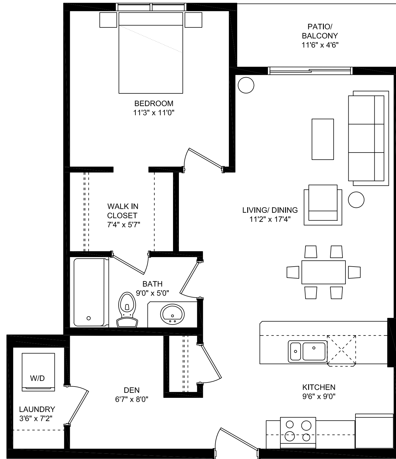
PLAN: UNIT B - 680 SFT Scale: 1/4" - 1'0"
