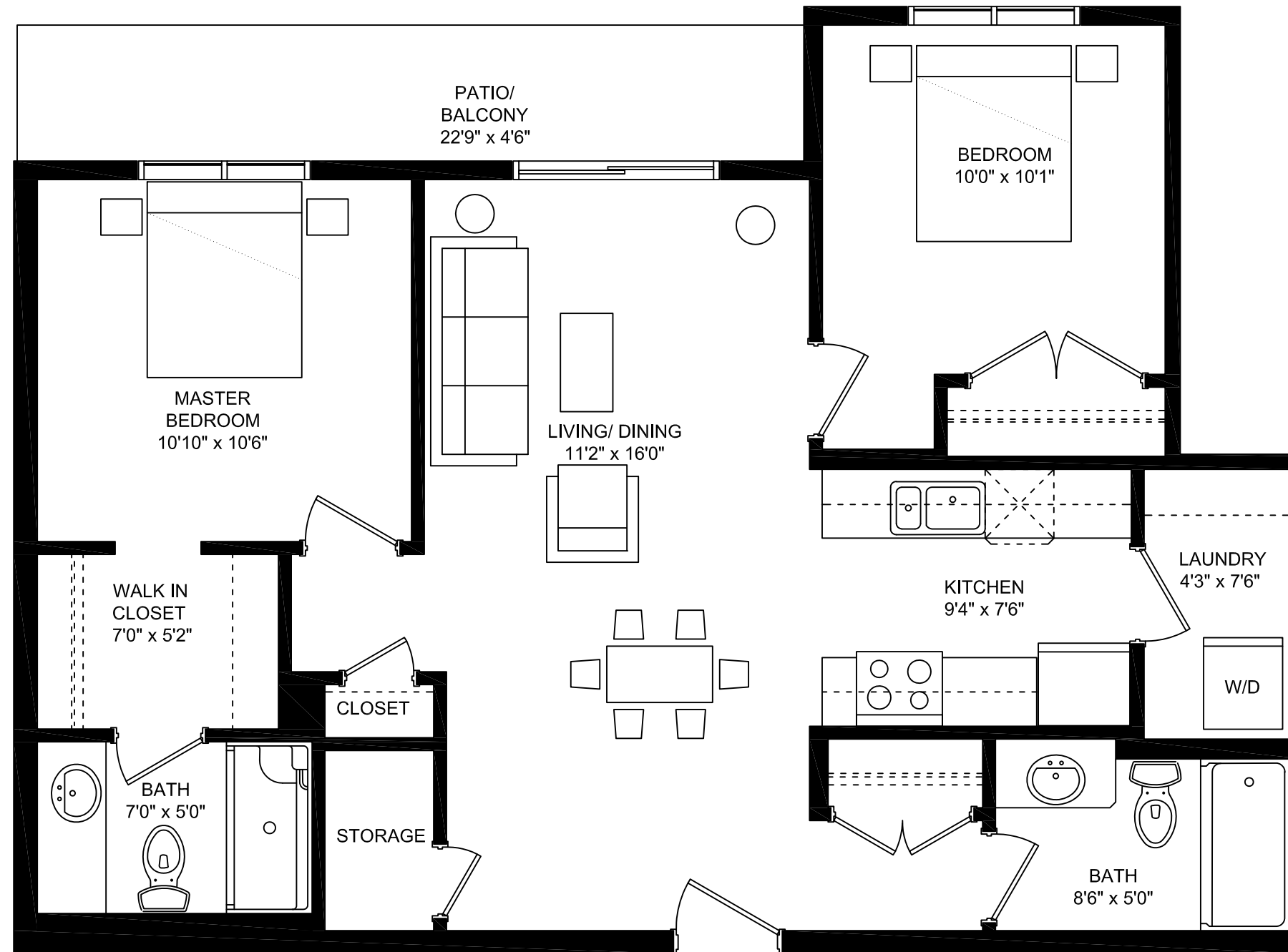
PLAN: UNIT C - 808 SFT Scale: 1/4" - 1'0"
