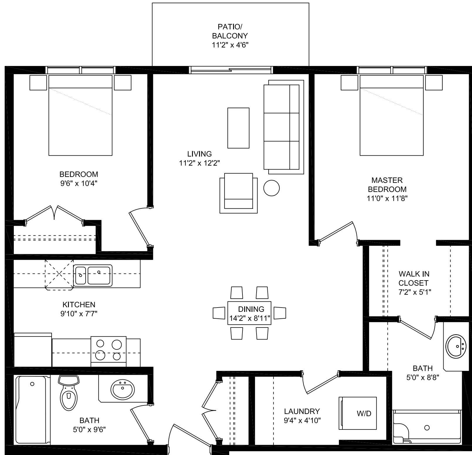
PLAN: UNIT H - 851 SFT Scale: 1/4" - 1'0"
